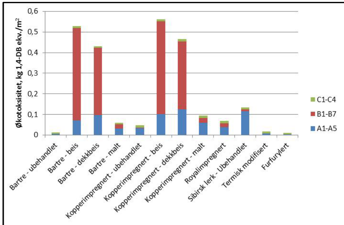
Figur 3. Utslipp av forbindelser som er giftige for vann- og jordlevende organismer. Figuren illustrerer utslipp relatert til behandlingsmetoder for trefasader. Den er hentet fra studien "Miljøanalyse av trefasader" som er utført som et samarbeid mellom SINTEF Byggeforsk, Treteknisk institutt og Norsk institutt for skog og landskap i Norge 21 . Faser A1-A5 inkluderer råvareutvinning, produksjon, installering av kledning inklusiv transport. Faser B1-B7 inkluderer bruksfasen (utslipp fra overflatebehandling og vedlikehold). Faser C1-C4 inkluderer riving og avfallsbehandling.
